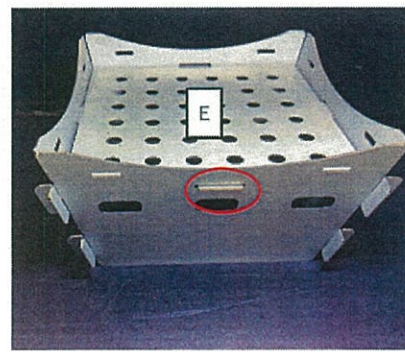
⑥部品Eを取り付ける
