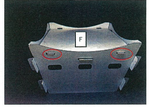
⑦部品Fを取り付ける
