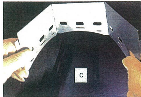
②部品Cを組み合わせる
