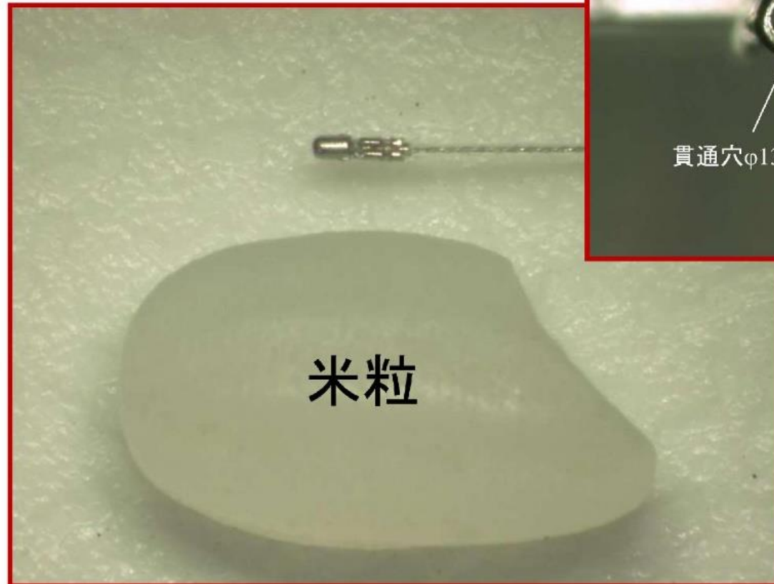
被覆径 \phi 0.1\text{mm} との圧着
