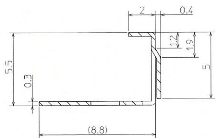
SEC. A-A
