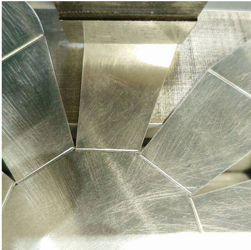
図6 手作業による曲げ加工
