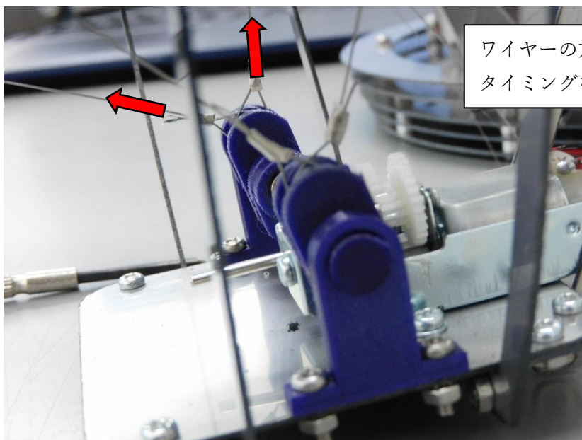
ワイヤーによる引張①
