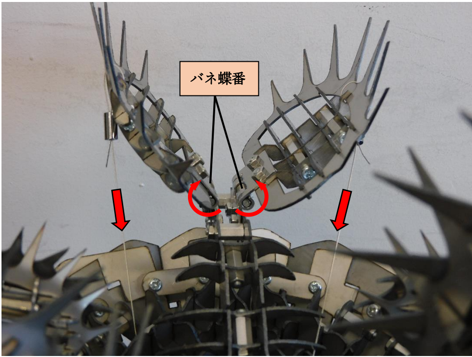
ワイヤーによる引張②
