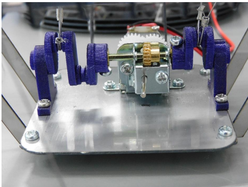
クランク機構
