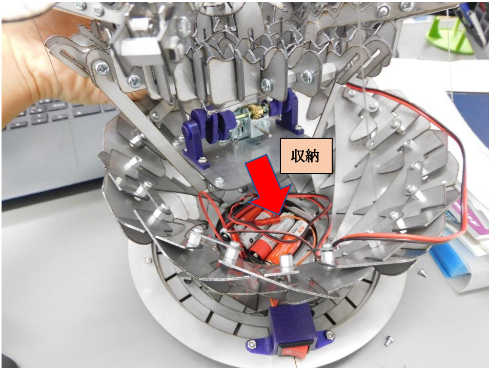
電動部品を内部に収納
