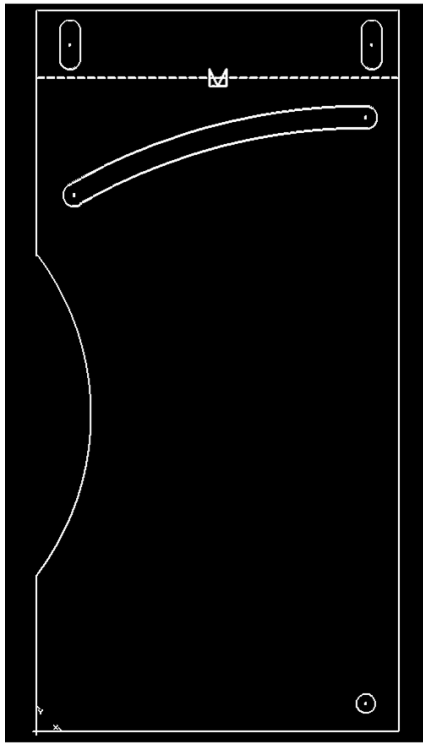
Fig.9 展開図 カバー2
