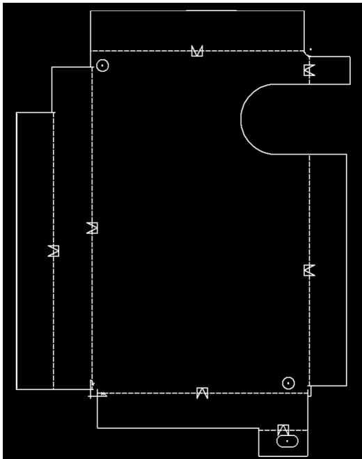
Fig.5 展開図 ケース
